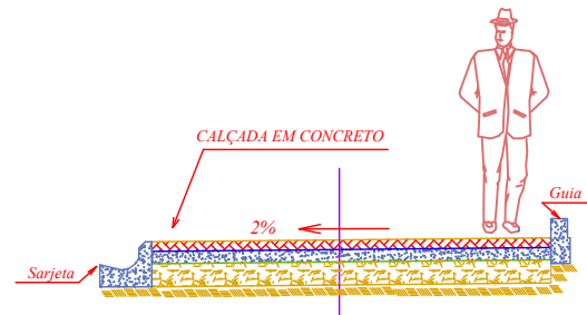
CORTE C - C Sem Escala
