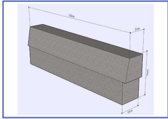
DETALHE 01: GUIA Sem Escala
