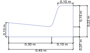
DETALHE 02: TRANSVERSAL DA GUIA E SARJETA Sem Escala
