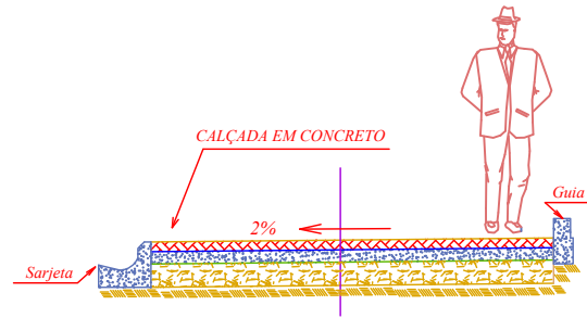
CORTE C - C Sem Escala
