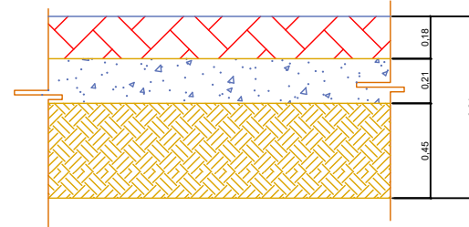
DETALHE 03: CALÇADA Sem Escala
