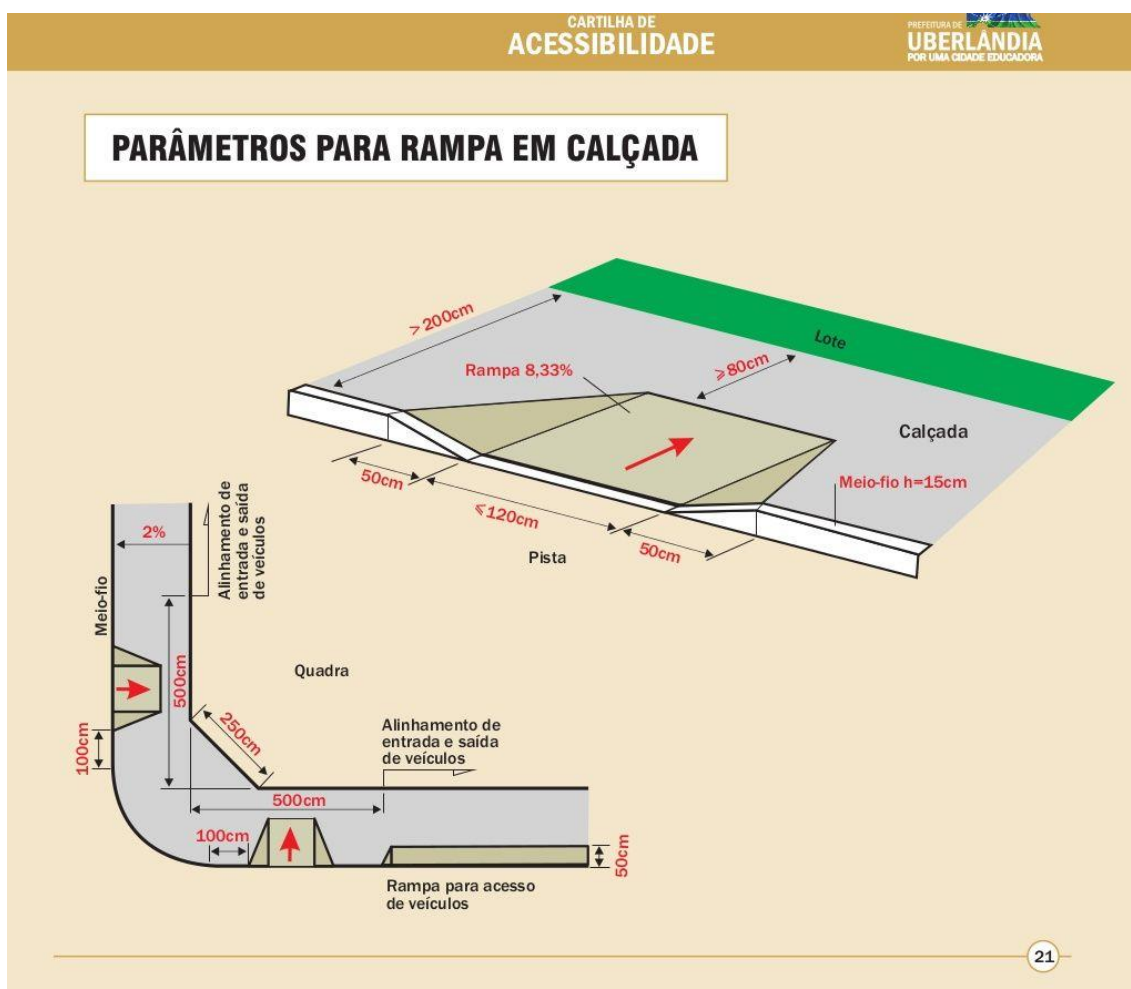
Figura 4 – Rebaixamento de Calçada e Acessibilidade
